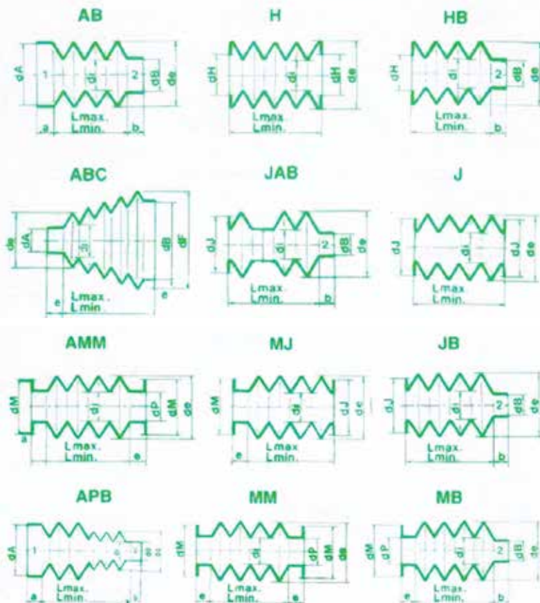
FCIJ harmonika méretei
